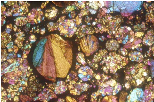
Typisches Gefüge eines chondritischen Meteoriten mit zahlreichen Schmelzkügelchen, sog. „Chondren“ (Bildbreite: ca. 4 mm).
