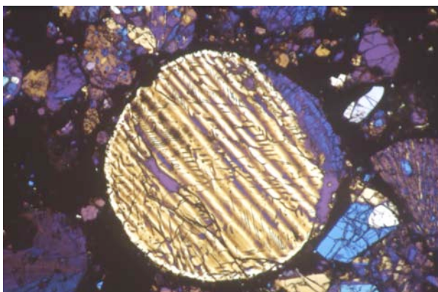
Balkenolvinchondre mit einem Durchmesser von ca. 700 µm, die seit ihrer Entstehung vor fast 4.6 Milliarden Jahren bis heute nahezu unverändert in dem Chondriten „Sharps“ vorliegt.
