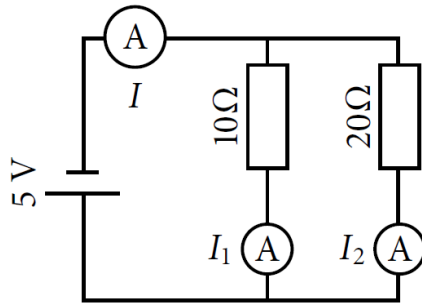
Schaltung a)
