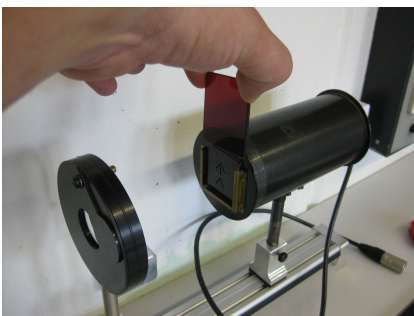
Abbildung 9.15: Haltevorrichtung für Farbfilter
