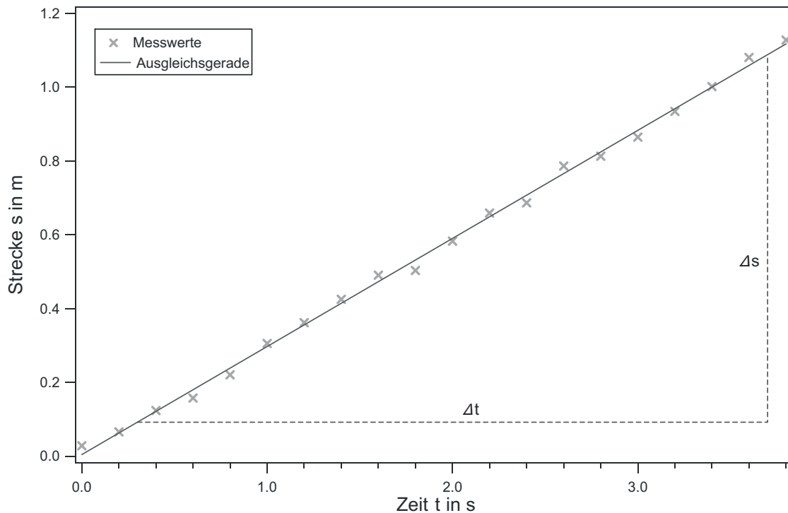
Abbildung II.3: Strecke aufgetragen gegen Zeit
