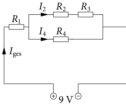
Abbildung 13.11: Kombinierte Schaltung
