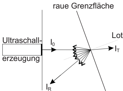
Abbildung 17.3: diffuse Streuung an rauher Oberfläche
