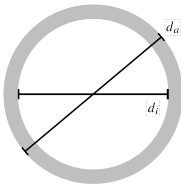
Abbildung 1.3: Die Grundfläche des Hohlzylinders (in der Abbildung grau dargestellt) ist die Differenz aus der Fläche des Außenkreises mit Durchmesser d_a und der Fläche des Innenkreises mit Durchmesser d_i .
