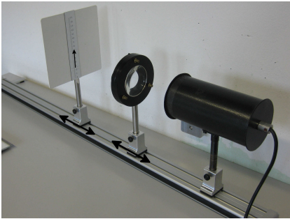
Abbildung 9.14: Optische Bank
