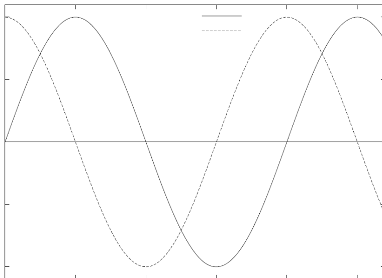
Abbildung III.5: Trigonometrische Funktionen
