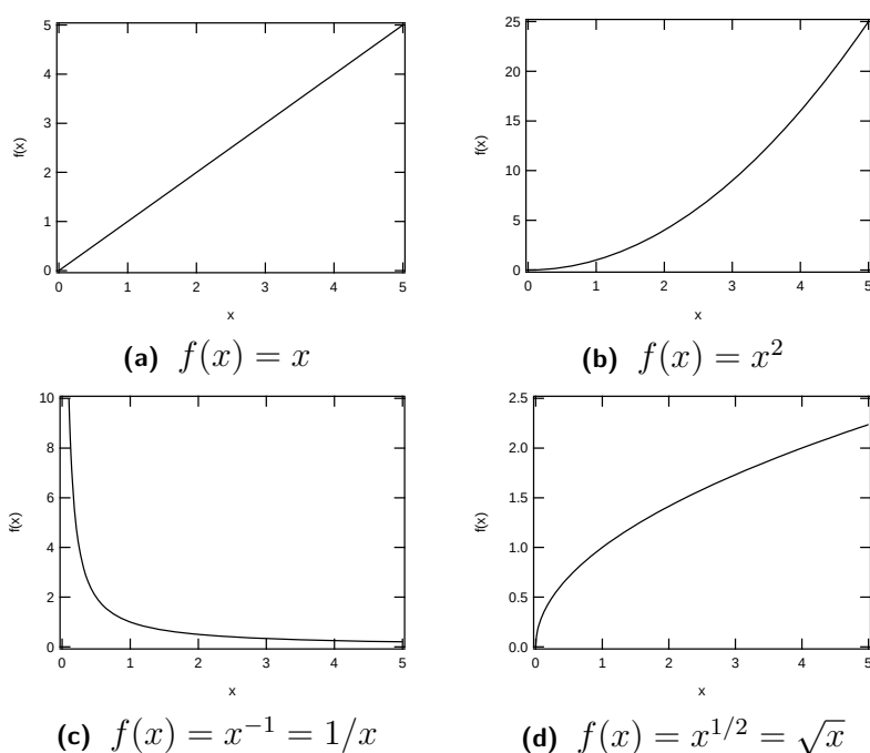
Abbildung III.1: Wichtige Potenzfunktionen
