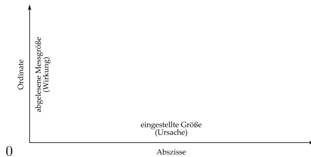
Abbildung II.1: Auftragung der Messgrößen in ein Diagramm
