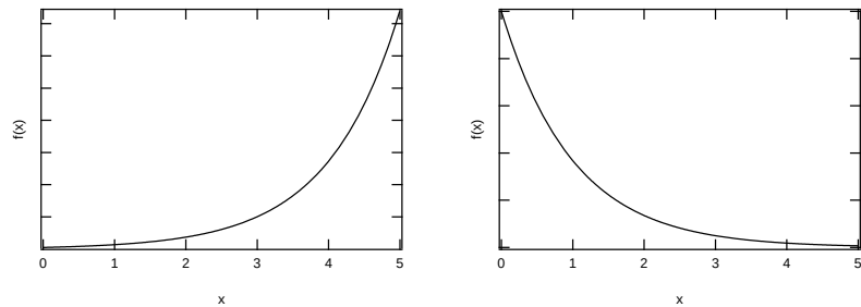
(a) Wachstumsfunktion ( b > 0 )
