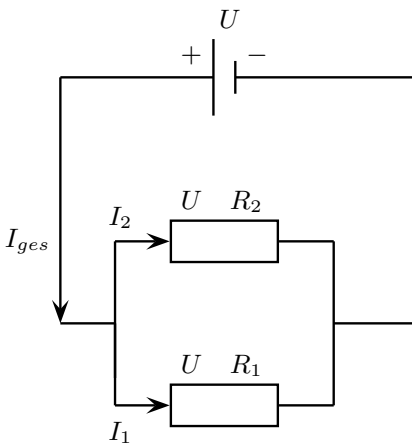
Abbildung 13.4: Parallelschaltung
