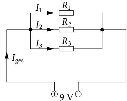
Abbildung 13.9: Parallelschaltung
