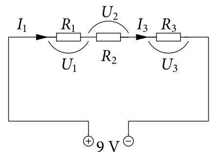
Abbildung 13.10: Reihenschaltung
