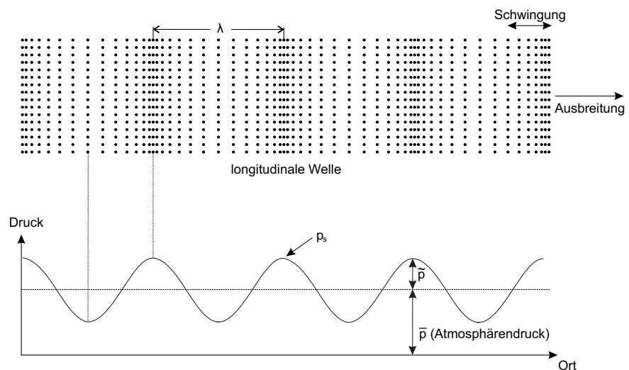
Abbildung 17.1: Ausbreitung von Schallwellen und die lokalen Druckunterschiede
