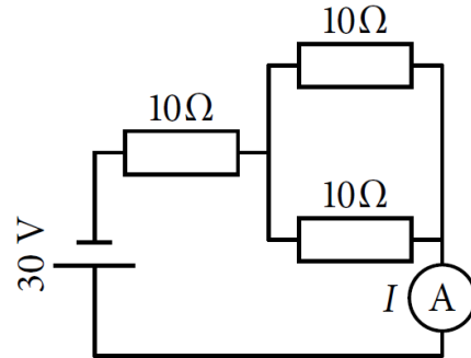
Schaltung b)
