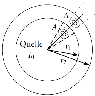
Abbildung 11.4: Abstandsgesetz: Die Quelle sendet eine Strahlung der Intensität I_0 aus. Misst man die Intensität I im Abstand r_1 und r_2 bei konstanter Fläche A , so gilt Gleichung 11.8
