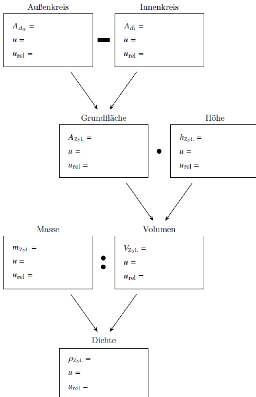
Abbildung 1.6: Diagramm zur Unsicherheitsfortpflanzung bei der Berechnung der Dichte des Hohlzylinders
