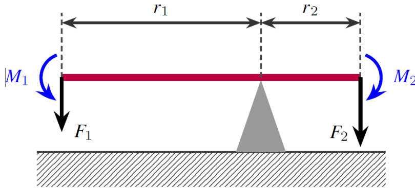
Abbildung 2.1: Skizze eines zweiseitigen Hebels im Gleichgewicht mit Hebelarmen r_1, r_2 , Kräften F_1, F_2 und den wirkenden Drehmomenten M_1, M_2 .
