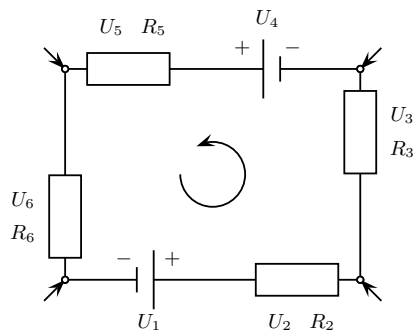
Abbildung 13.3: Maschenregel
