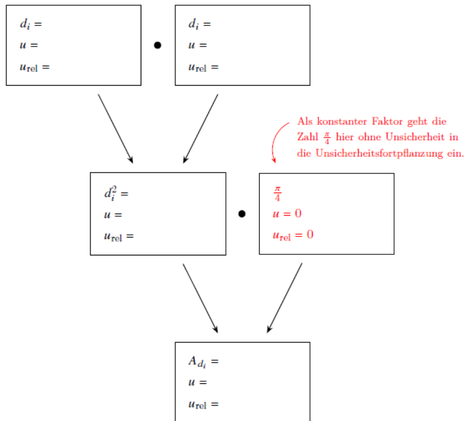
Abbildung 1.5: Diagramm zur Unsicherheitsfortpflanzung bei der Berechnung der Innenkreisfläche
