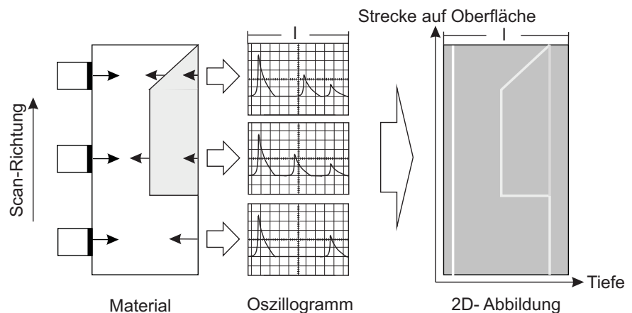
Abbildung 17.6: Erzeugung eines 2D-Ultraschallbildes (B-Mode)
