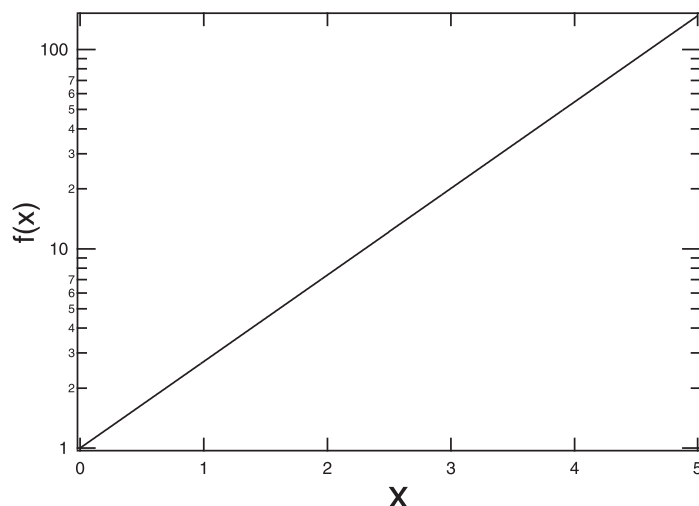
Abbildung III.4: Halblogarithmische Darstellung einer Exponentialfunktion
