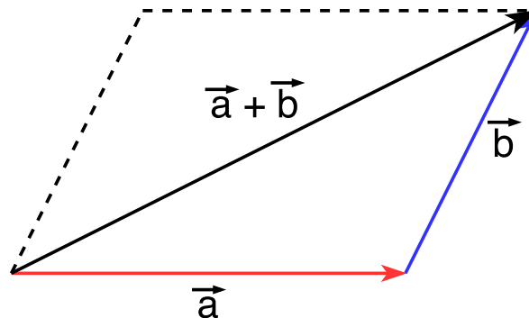
Abbildung III.8: Addition von Vektoren
