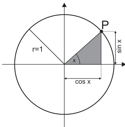
Abbildung III.6: Einheitskreis
