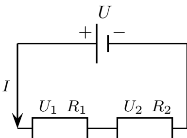
Abbildung 13.5: Reihenschaltung
