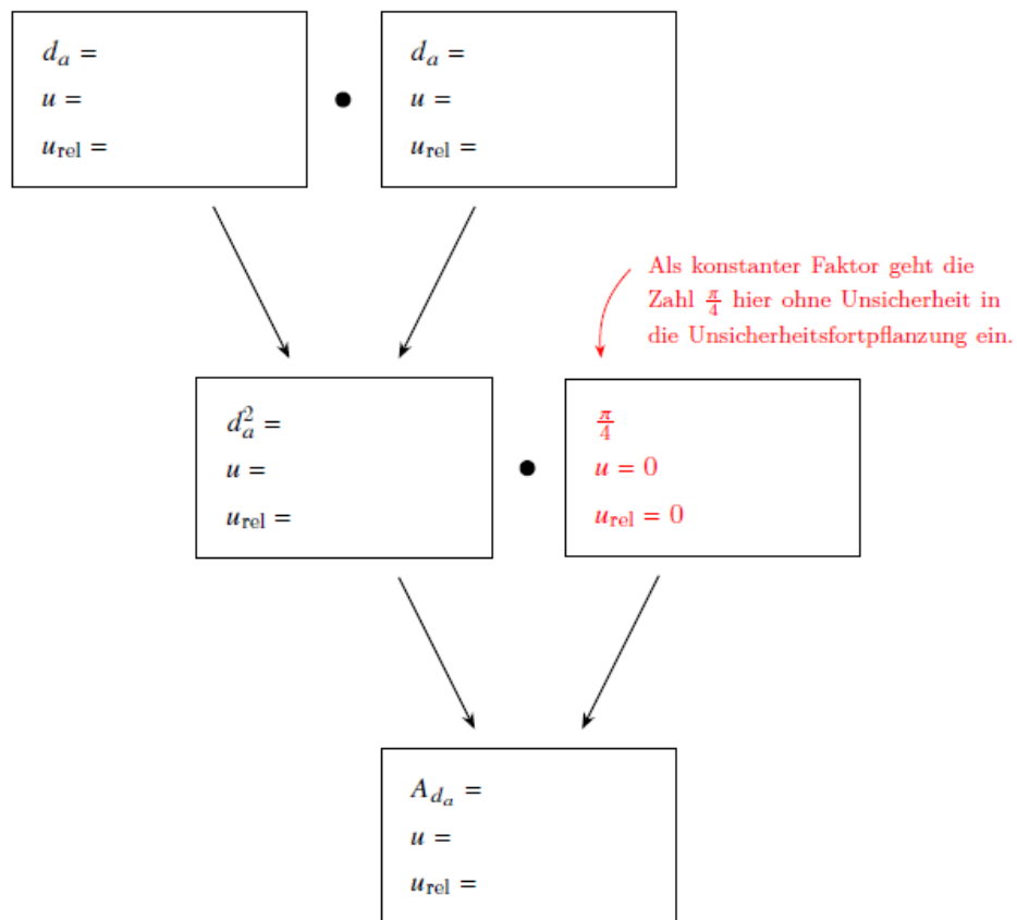
Abbildung 1.4: Diagramm zur Unsicherheitsfortpflanzung bei der Berechnung der Außenkreisfläche
