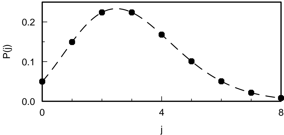
Poisson-Verteilung für \lambda=3
