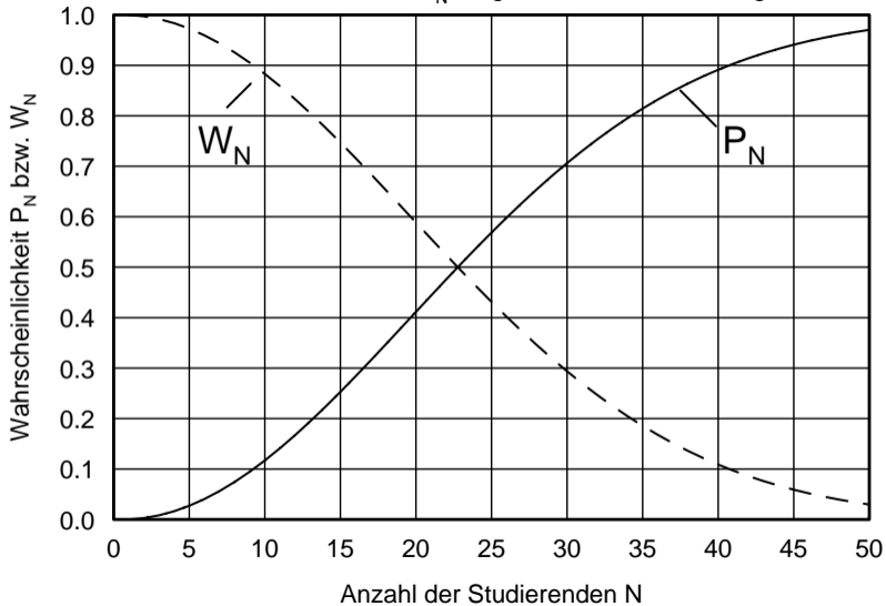
Wahrscheinlichkeit P_N für gemeinsame Geburtstage
