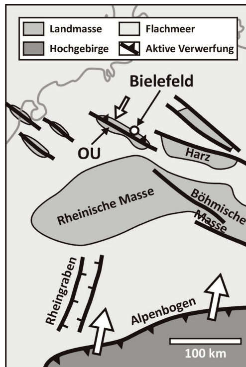
Abb. 4: Deutschland in der jüngsten Kreidezeit vor 70 Millionen Jahren (nach ZIEGLER 1990). Die Pfeile deuten Bewegungsrichtungen der Erdkruste an, wie sie seinerzeit geherrscht haben (nach Sippel et al. 2009). OU = Osning-Überschiebung.
