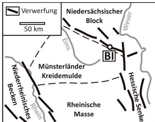
Abb. 5: Tektonischer Bau im Untergrund von Norddeutschland (verändert nach KRONBERG 1991 und VOGT & GRÜNTAL 1994). Die Grenzen zwischen den einzelnen Schollen sind durch tief reichende Verwerfungen in der Erdkruste markiert. Die Rheinische Masse setzt sich unterhalb der Münsterländer Kreidemulde fort, ist dort aber von mächtigen Sedimentgesteinen überdeckt, die sich im kreidezeitlichen Flachmeer abgelagert haben.
