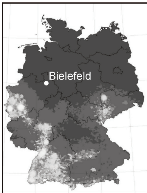
Abb. 3: Erdbebenrisiko-Karte für Deutschland aus THIEKEN et al. (2007). Hellere Töne bedeuten im Wesentlichen höhere Erdbebenhäufigkeit und damit höhere Wahrscheinlichkeit von Erdbebenschäden. Bielefeld liegt in einem Gebiet, in dem Erdbeben höchst selten sind.
