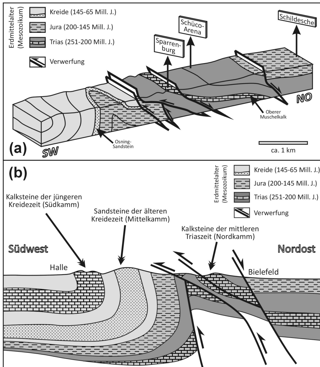
Abb. 6: (a) Schnitt durch den Untergrund des Bielefelder Stadtgebiets, basierend auf MESTWERTD & BURRE (1981). Die Sparrenburg steht auf triaszeitlichen Kalksteinen, die vor 70 Millionen Jahren über die eigentlich jüngeren Gesteine der Jura- und Kreidezeit geschoben wurden. Eine dieser alten Überschiebungsbahnen ist sehr wahrscheinlich im Jahre 1612 erneut in Bewegung geraten. (b) Schnitt durch den Kamm des Teutoburger Waldes, nach der Geologischen Karte 1:100.000, Blatt Bielefeld (1986). Die triaszeitlichen Kalksteine (240 Millionen Jahre alt), sowie der unterkreidezeitliche Osning-Sandstein (120 Millionen Jahre alt) und die Kalksteine der Oberkreide (90 Millionen Jahre alt) sind sehr verwitterungsbeständig. Sie bilden daher heute die schmalen Kämmе des Teutoburger Waldes. Man beachte die starke Verbiegung der Schichten durch die Osning-Überschiebung, die im südlichen Bereich des Kamms sogar überkippt stehen (vergleiche auch Abb. 7).
