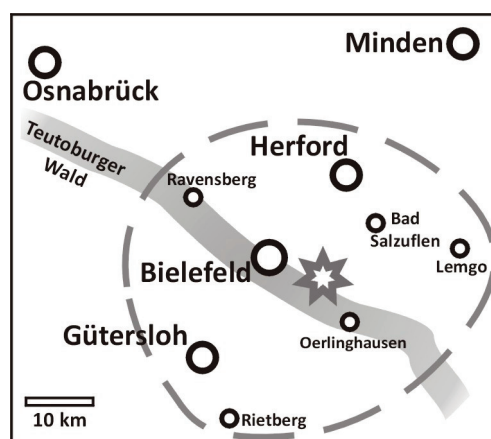
Abb. 2: Wahrscheinliches Epizentrum und Wirkungsbereich des Bebens von 1612 (nach VOGT & GRÜNTAL 1994). Die gestrichelte Linie umfaßt die Orte, in denen das Beben dokumentiert worden ist.
