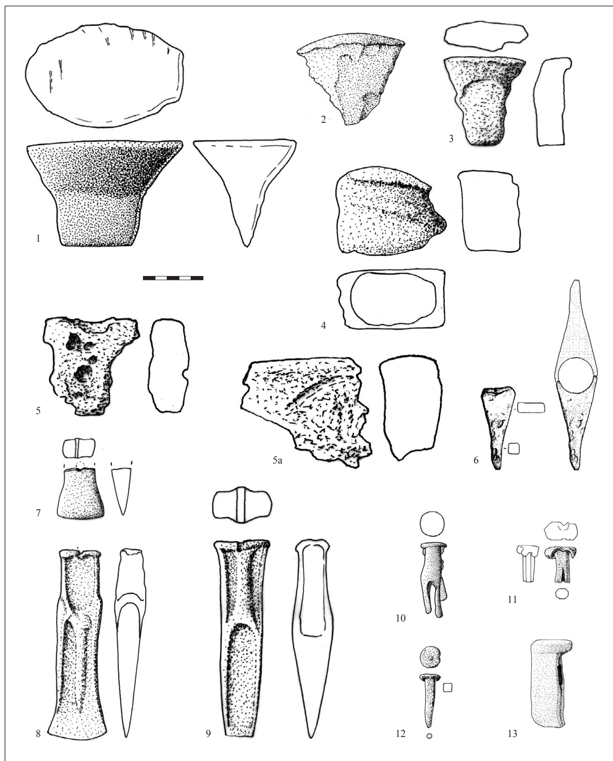
Fig. 16. Ad-hoc- anvils: 1) Pontpoint (no. 41); 2) Jarpice (no. 7); 3) Gușterița (no. 103); 4) Maintal-Hochstadt (no. 53); 5, 5a) Oberwilfingen (no. 56); 6) Lachen-Speyerdorf (no. 52); 7) Damsholte (no. 17); 8) Bromma (no. 106); 9) Holmedal (no. 107); 10) Nantes-Prairie de Mauves (no. 37); 11) Bologna-San Francesco (no. 81); 12) Redù (no. 88); 13) Augsdorf (no. 1). – Bronze. – M. 1:3
