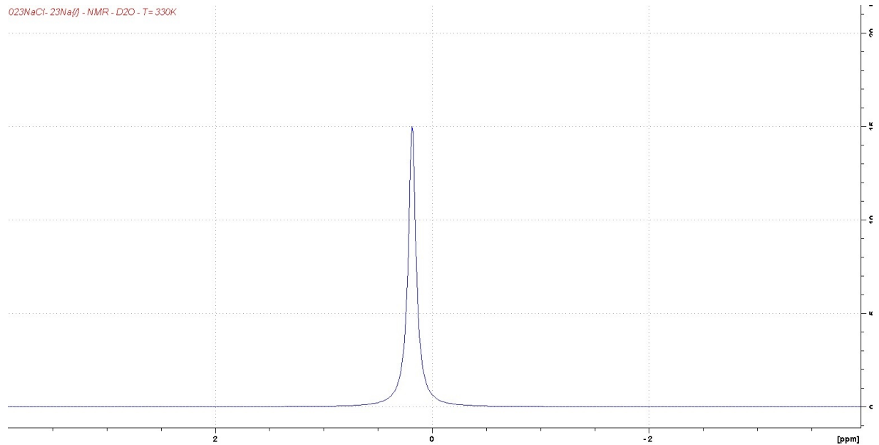
Abb. ^{23}\text{Na} -Spektrum
