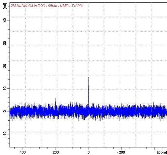
Abb. 95 Mo-Spektrum
