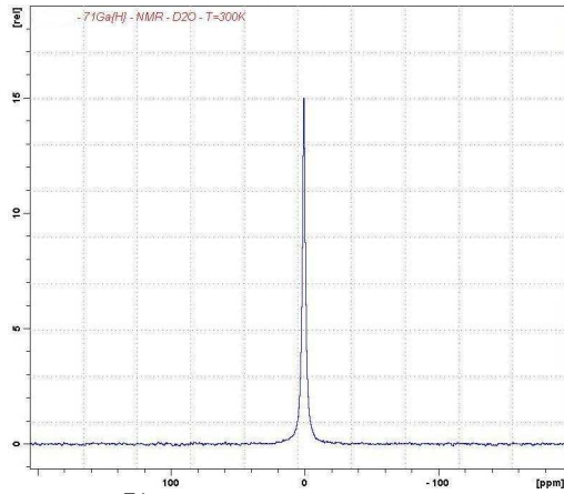
Abb. ^{71}\text{Ga} -Spektrum
