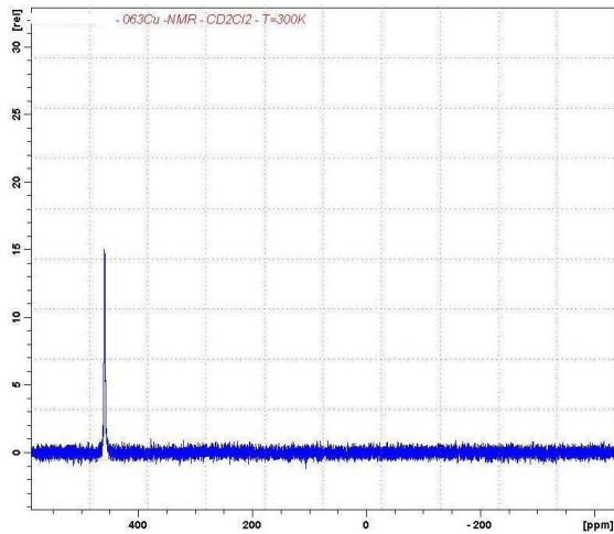
Abb. ^{63}\text{Cu} -Spektrum
