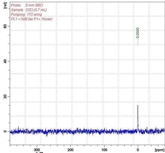
Abb. ^{17}\text{O} -Spektrum
