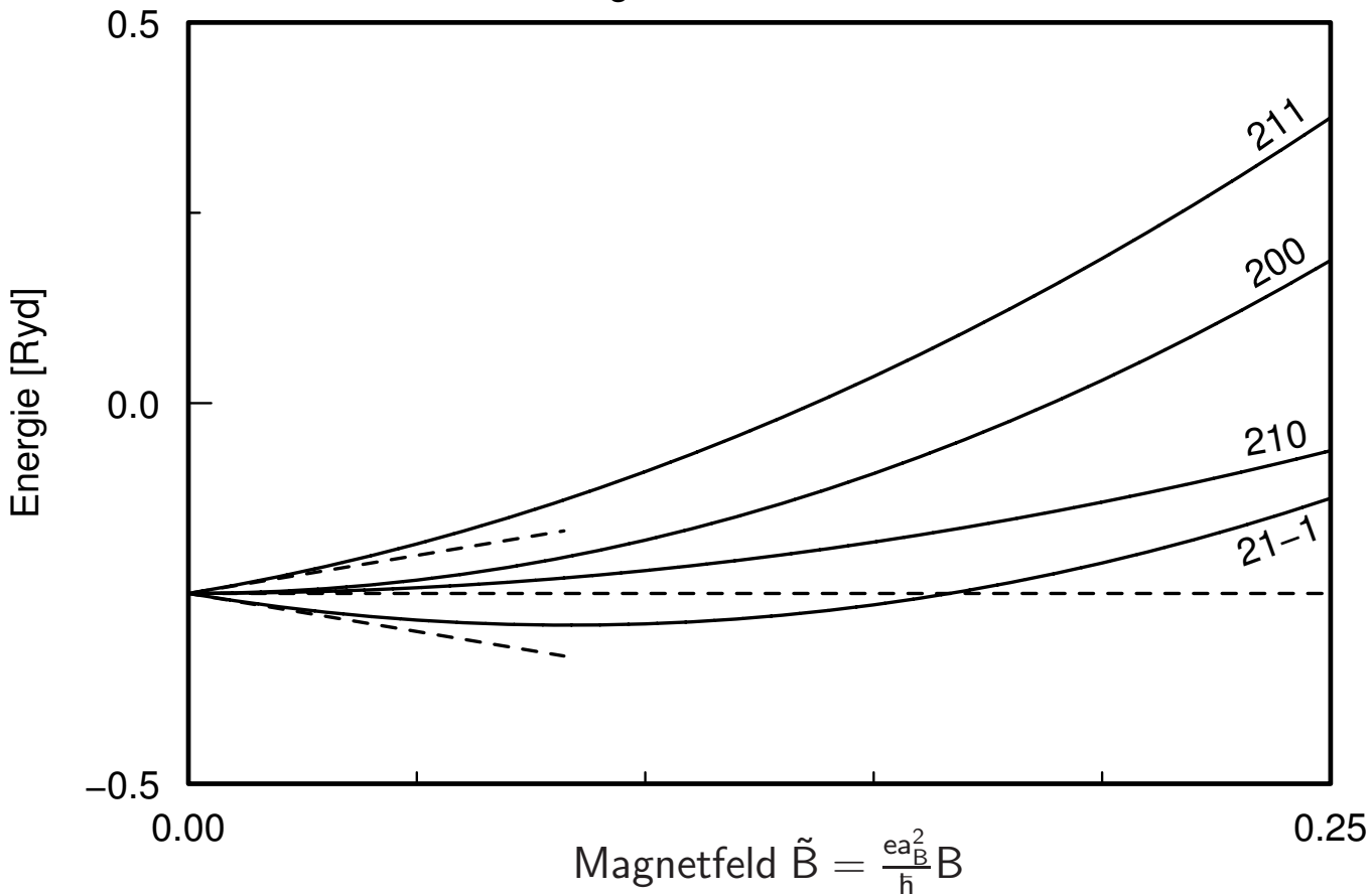
Energien der n=2 Zustände
