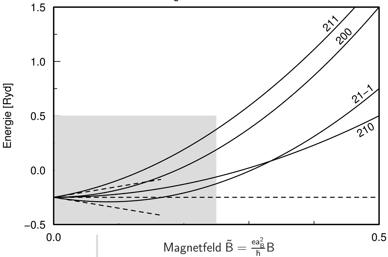
Energien der n=2 Zustände
