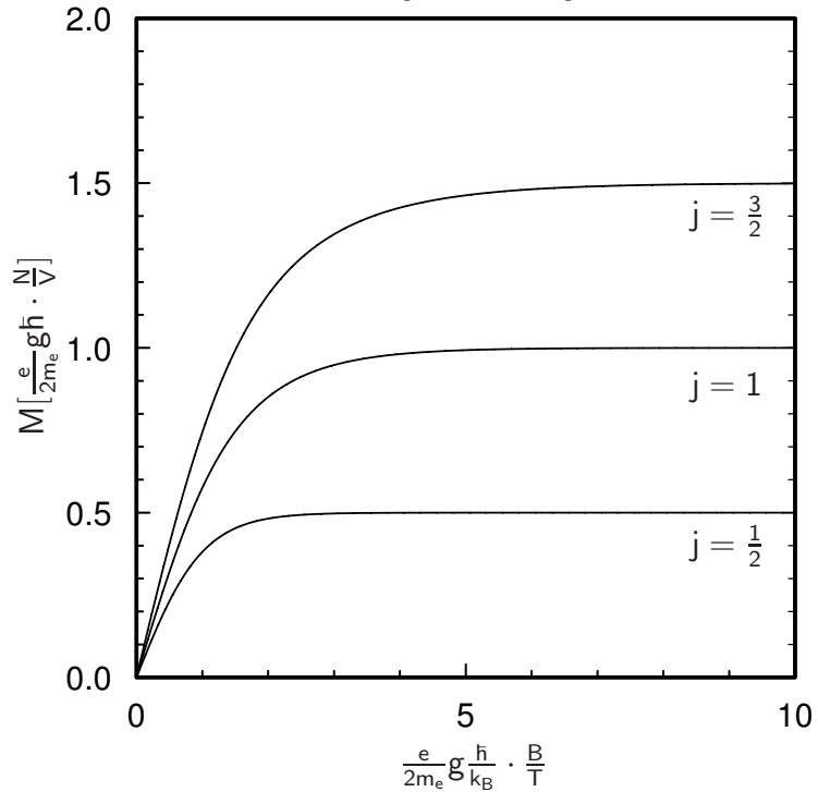
Magnetisierung
