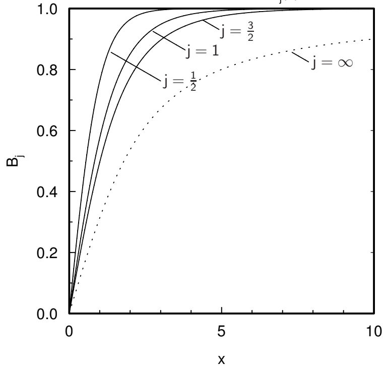
Brillouin-Funktion B_j(x)
