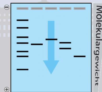
Prinzip der Gelelektrophorese
